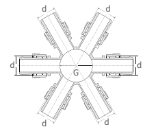
YÜZÜKLÜ YASSI ÇOKLU DAĞITIM NİPELİ TAPE (WITH RING) MULTICOUPLING NIPPLE
