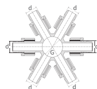
YASSI DAMLAMA ÇOKLU DAĞITIM NİPELİ DRIP TAPE MULTICOUPLING NIPPLE
