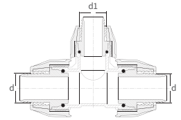
REDÜKSİYON TE REDUCING TEE
